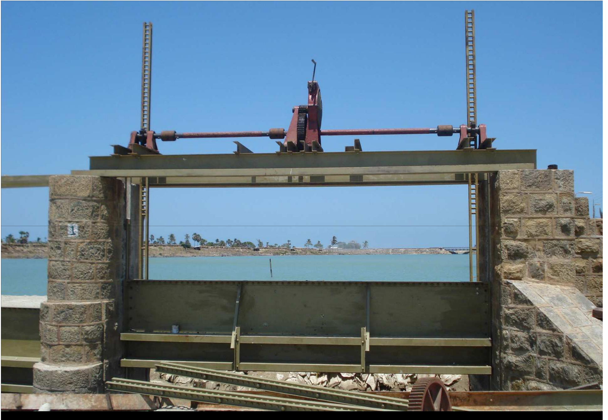
THONDAMANARU BARRAGE
